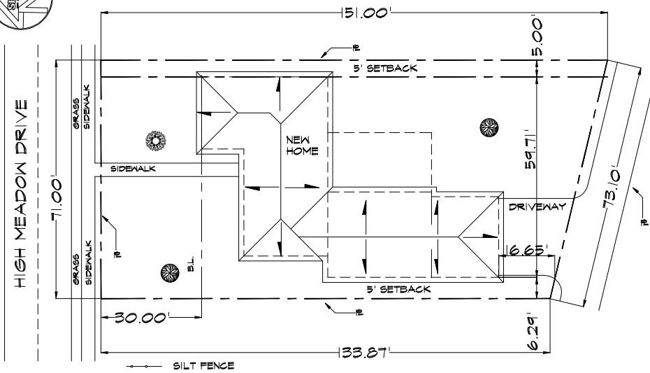
SITE PLAN SCALE: 1" = 20'
